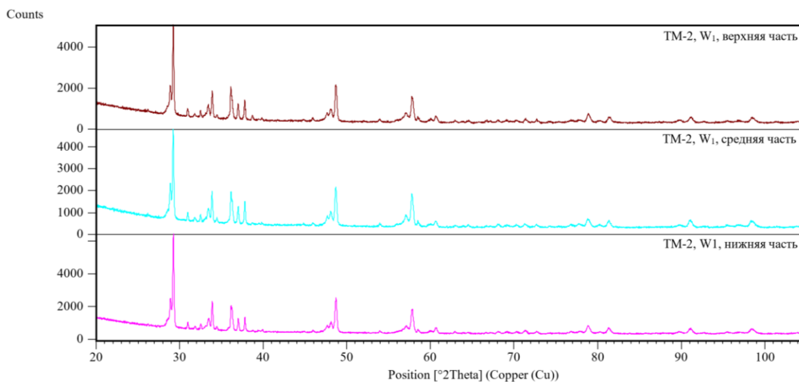
Рисунок 48 - Результаты фазового анализа слитка
