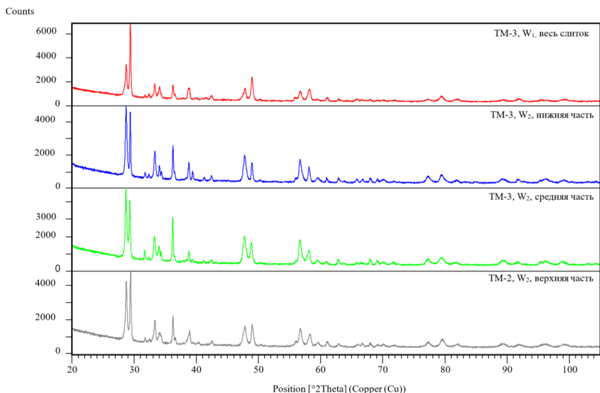
Рисунок 53 - Результаты фазового анализа слитков
