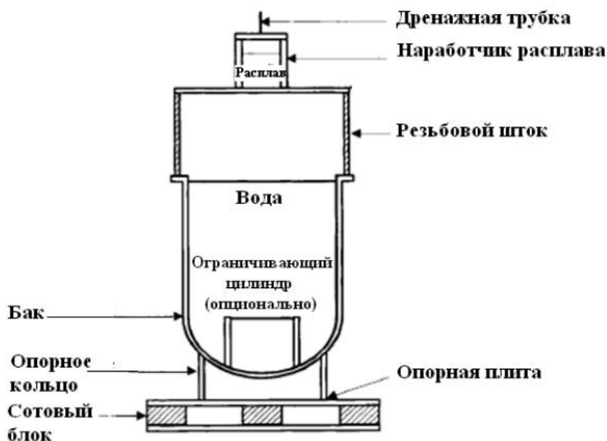
Рисунок 6 – Экспериментальная установка для проведения исследований паровых взрывов в открытой геометрии [47]
