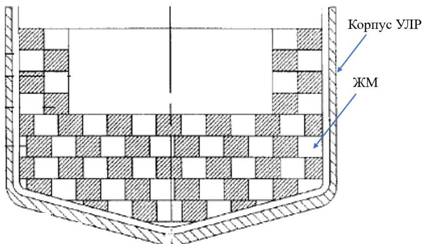
Рисунок 17 – Принципиальная схема УЛР реактора ВВЭР
