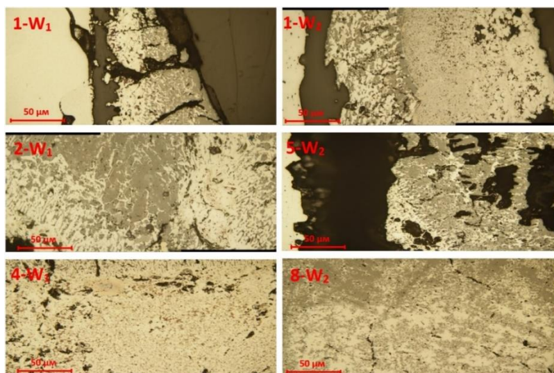
Рисунок 50 - Микроструктуры диаметральных разрезов слитков
