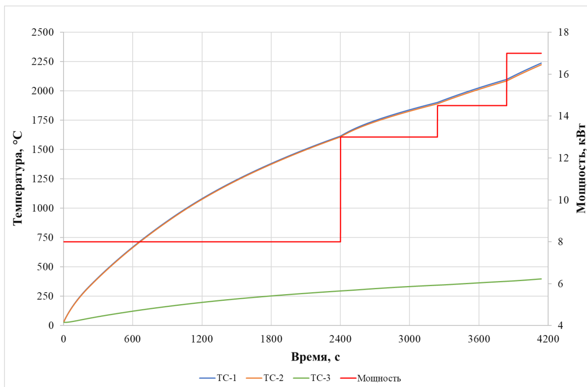
Рисунок 31 – Диаграмма нагрева графитового тигля
