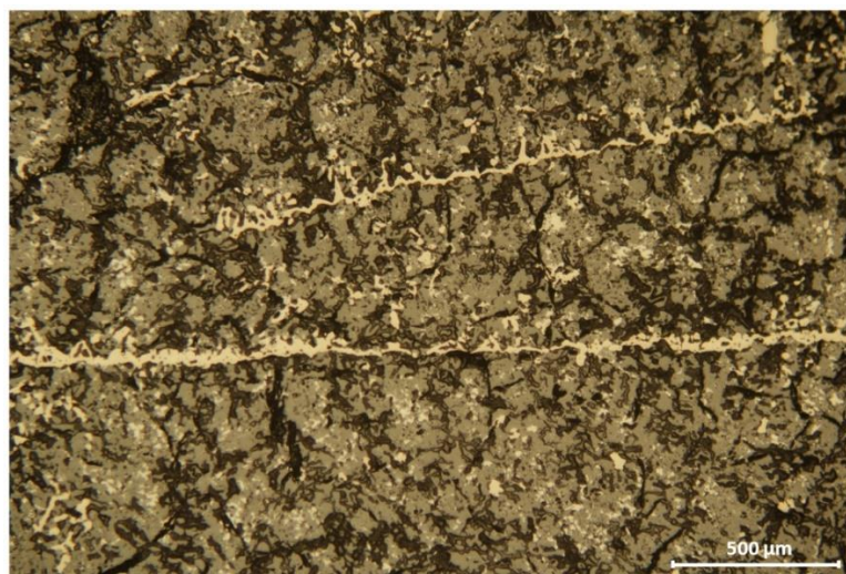
Рисунок 46 – Микроструктура кориума в области 4
