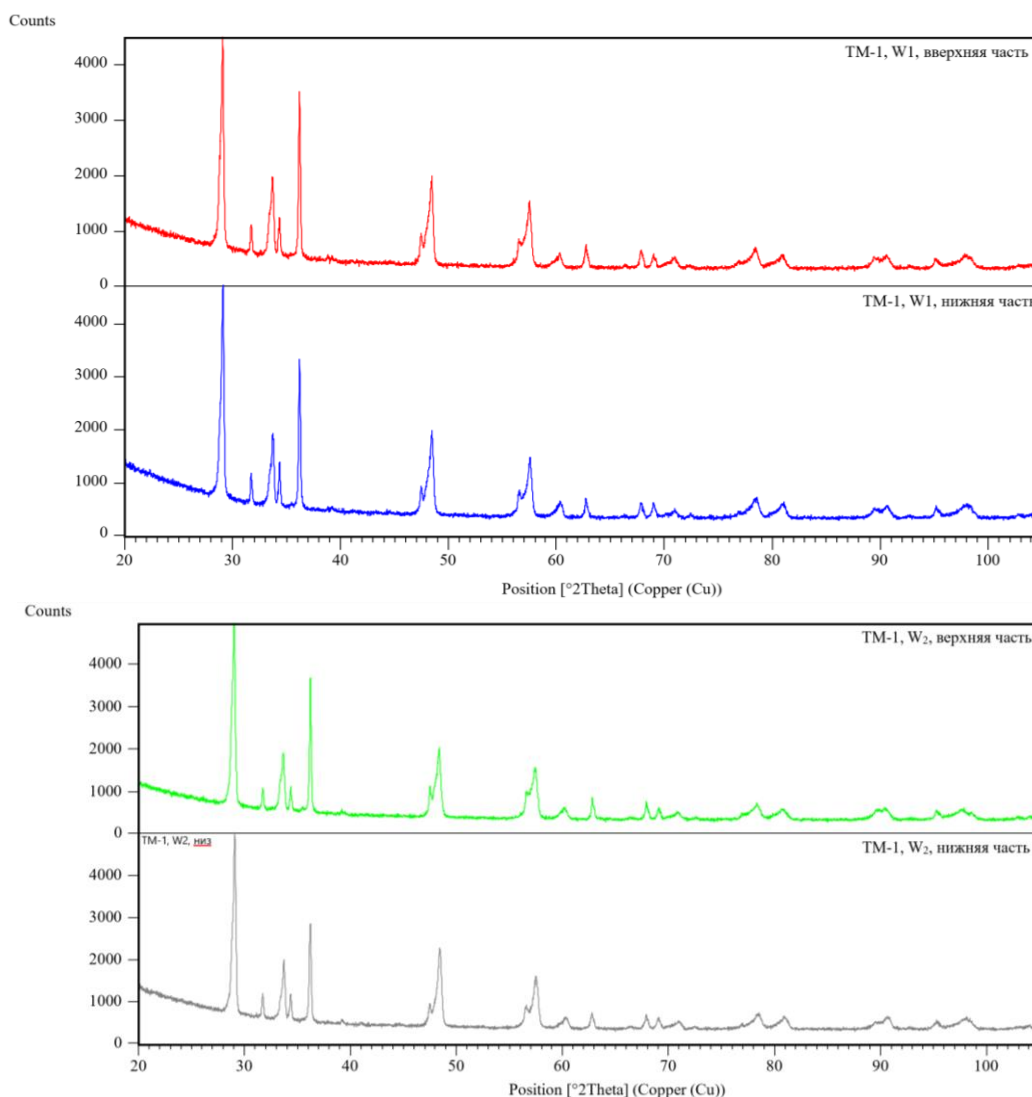
Рисунок 43 - Результаты фазового анализа слитков
