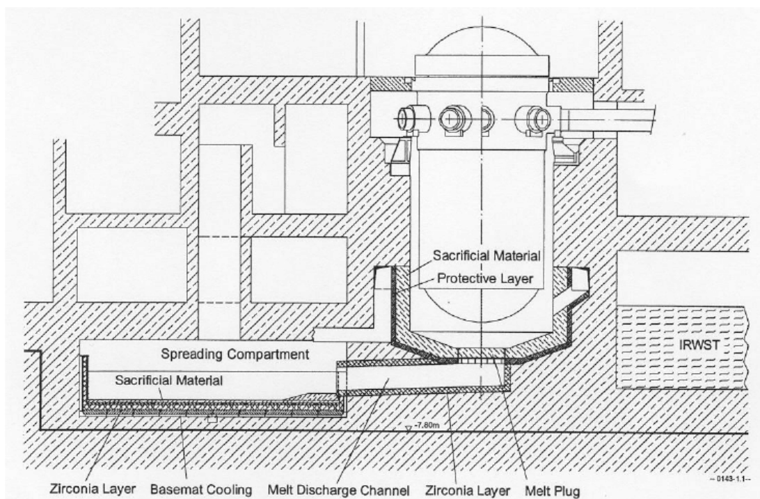
Рисунок 2 – Основные компоненты устройства локализации расплава реактора EPR [32]
