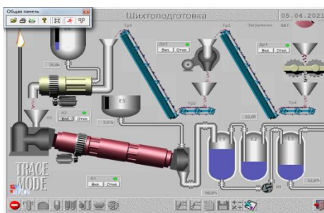
Рисунок 1 – Система, включающая полную диспетчеризацию и дистанционный контроль управления всеми исполнительными механизмами
