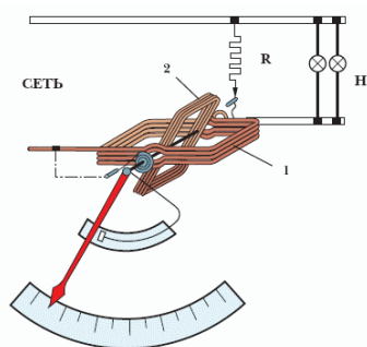
Рисунок 1 – Принцип действия ваттметра
