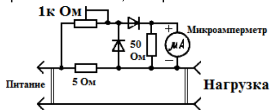
Рисунок 2 – Электрическая схема прибора
